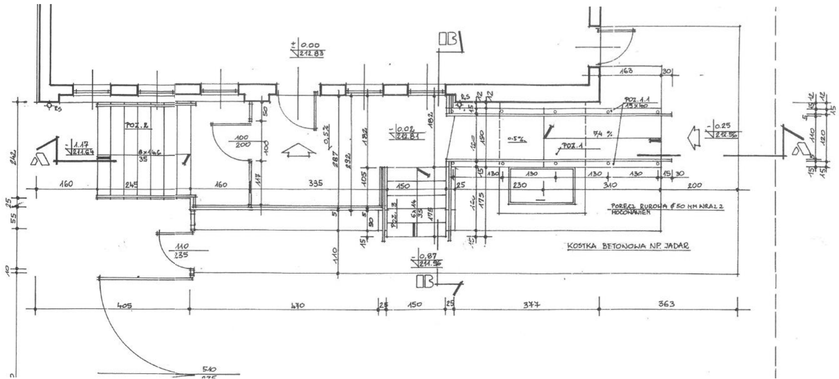
Rzut Przyziemia – stan istniejący
