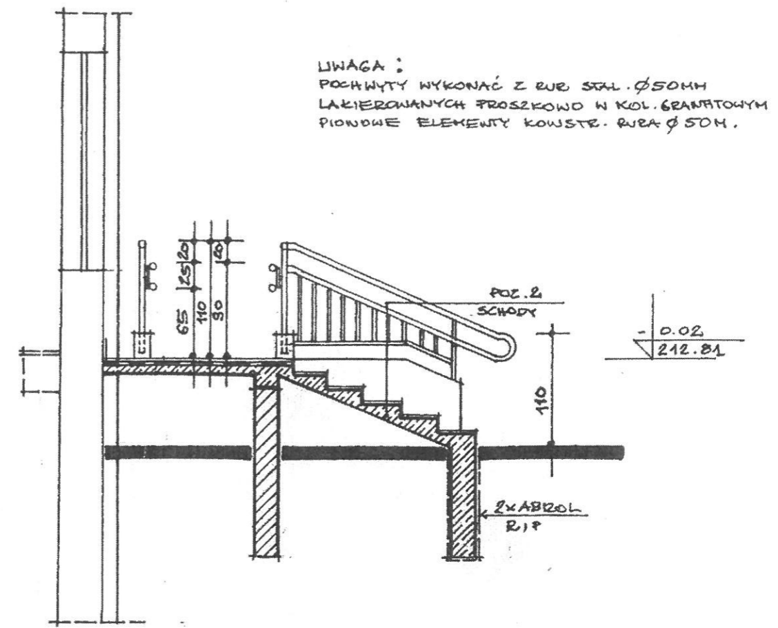
poz. 2 schody 03 - 03
